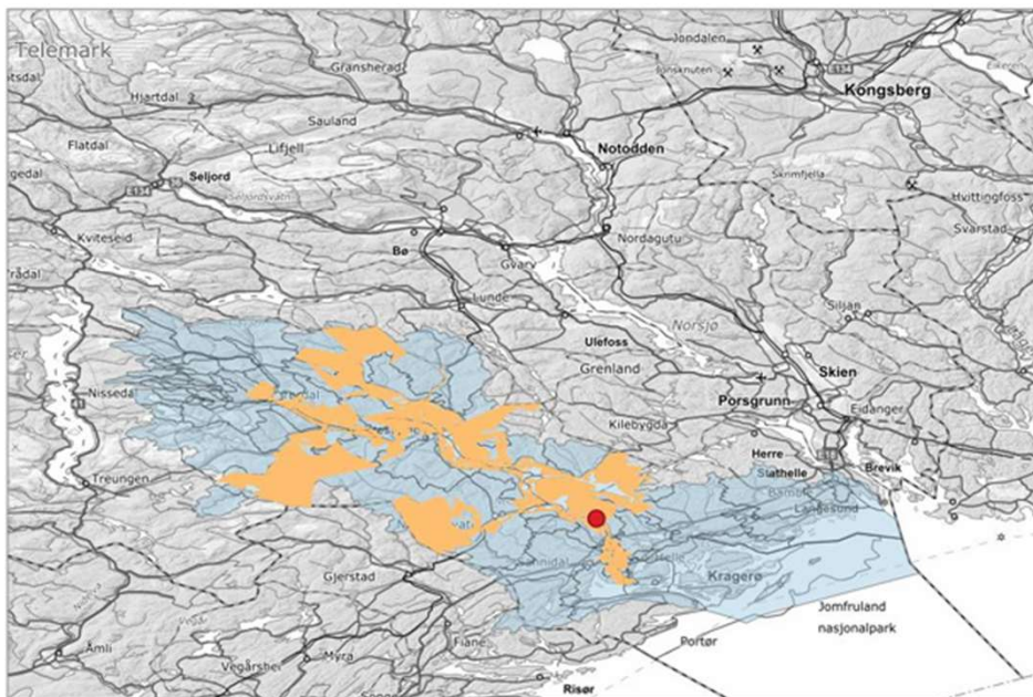
Figur: Eiendommer som grenser til Kragerøvassdraget (oransje), nedbørfelt (blått) og lokalisering av Dalsfos kraftverk (rød prikk).
